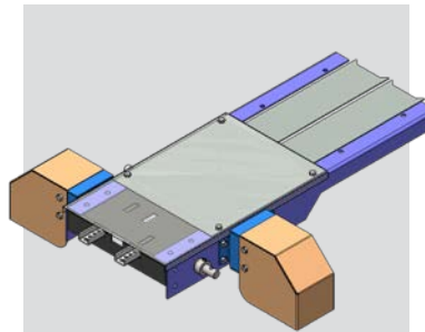
ACCIONADORES DE LA CORREDERA DE LA BOTA
